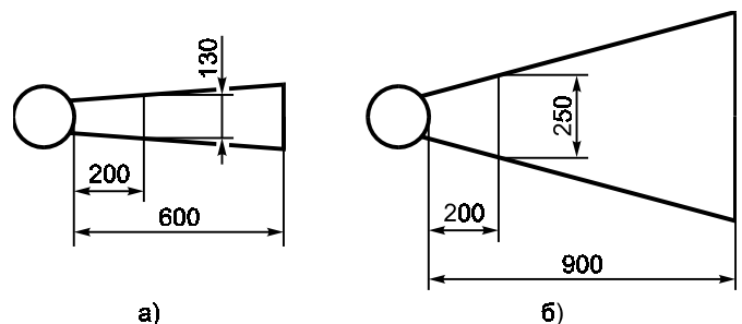
Рисунок 2 — Размеры спиральных и винтовых лестниц
